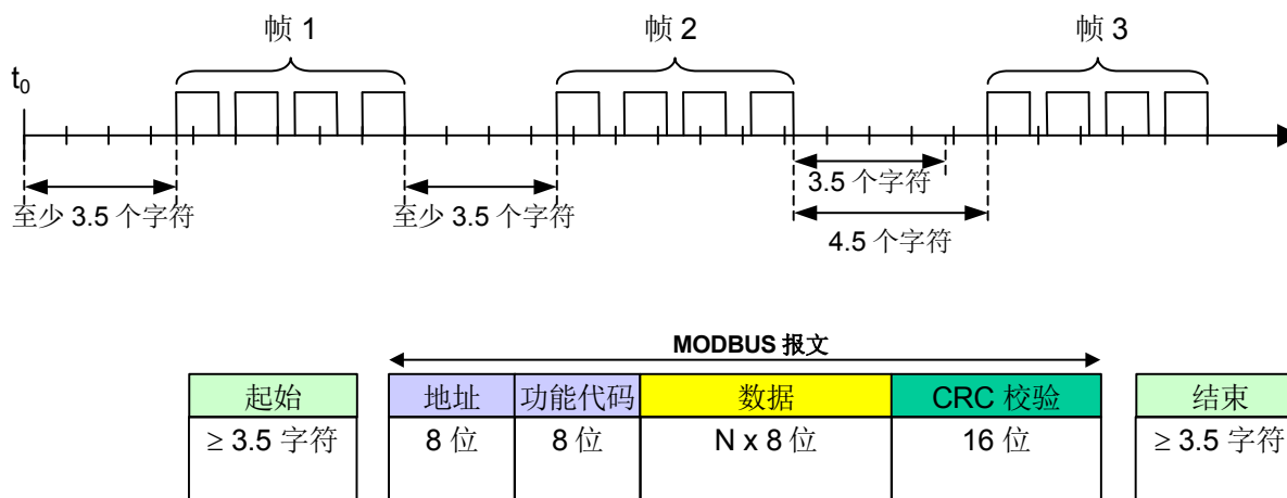
图 10: RTU 报文帧
